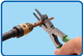
Deșurubarea duzei
